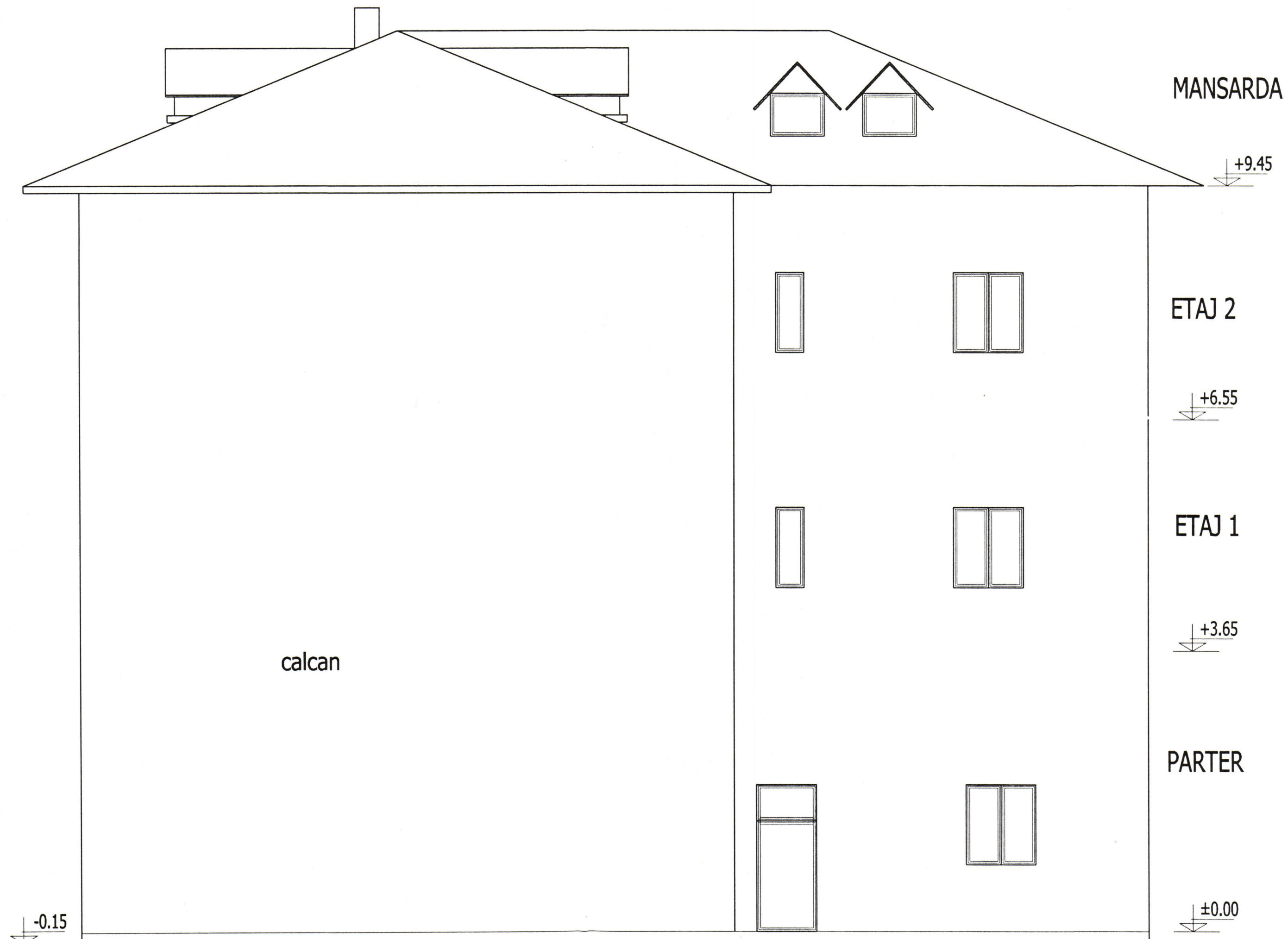
FATADA LATERALA DREAPTA
